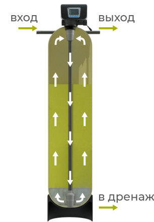
1. Обратная промывка
