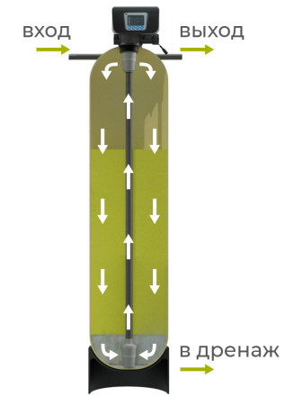
2. Прямая промывка
