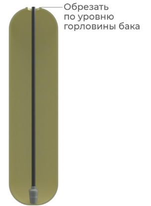
Обрезка водоподъемной трубы
